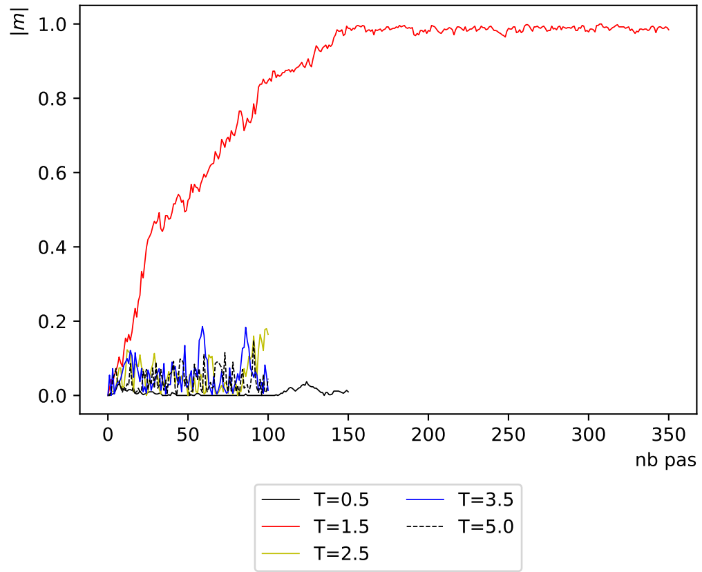
Evolution selon critère Estimation par intervalle,Condition Initiale alterné 4lignes-4lignes, Réseau taille L=32
